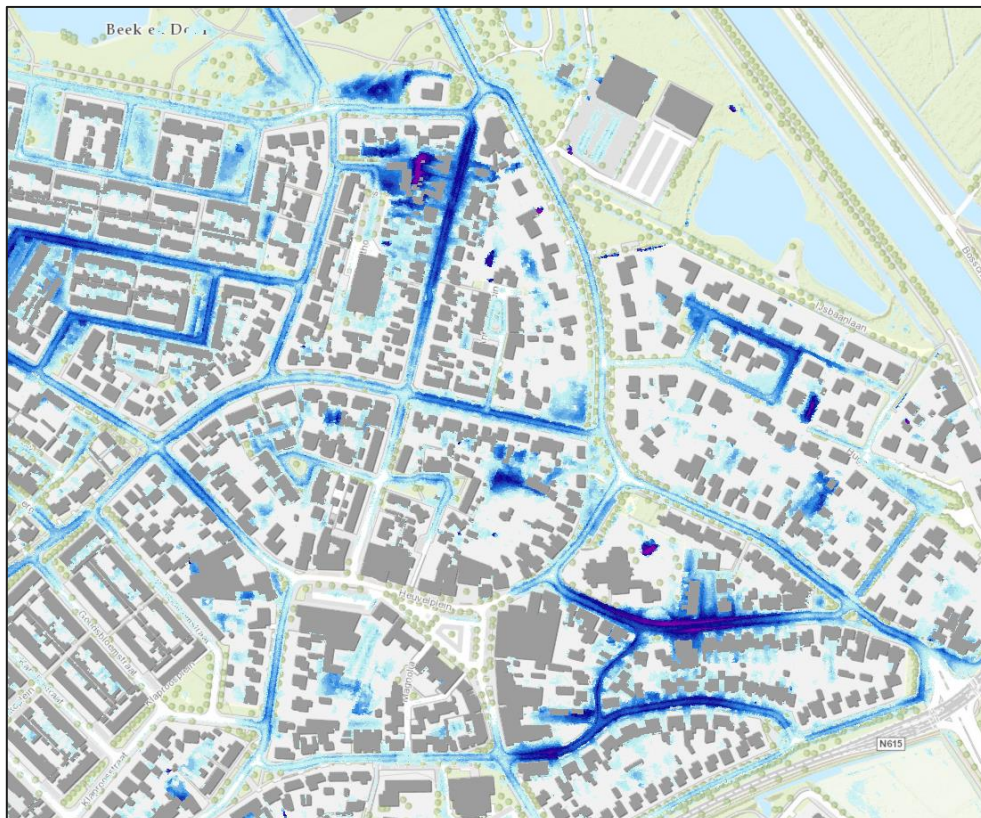
Figuur 3 - Resultaat uit de hydraulische simulatie van water op straat in Beek en Donk (70 mm in 1 uur).
