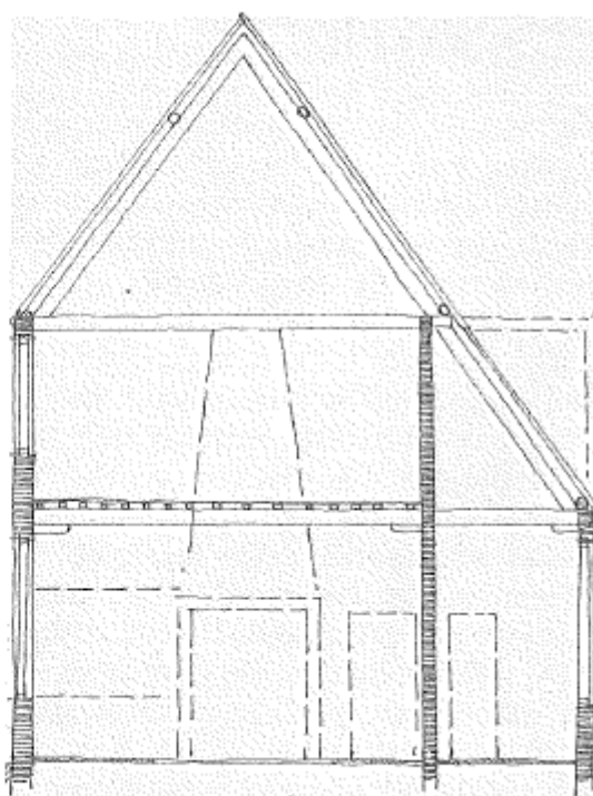
16. Aarle-Rixtel, Havenweg 1-3, dwarsdoorsnede, schets. Tekening van P. Ingen-Housz, 1979.
